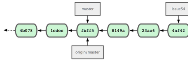
Рисунок 5.7: Исходная история коммитов Джессики.
