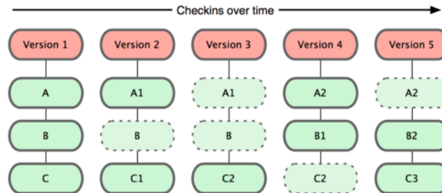
Рисунок 1.5: Git хранит данные как слепки состояний проекта во времени.
