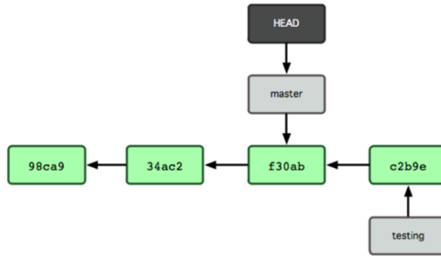
Рисунок 3.8: HEAD перемещается на другую ветку при checkout'е.
