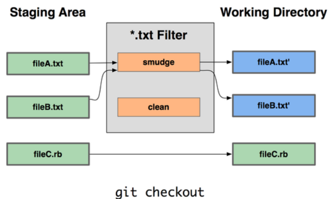
Рисунок 7.2: Фильтр «smudge» выполняется при checkout.
