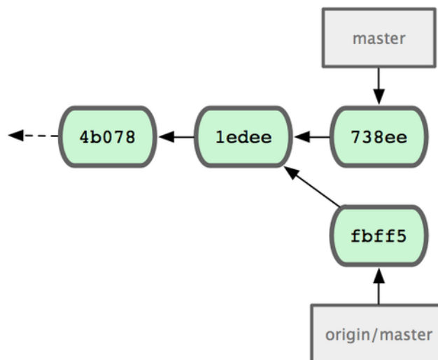
Рисунок 5.4: Исходный репозиторий Джона.
